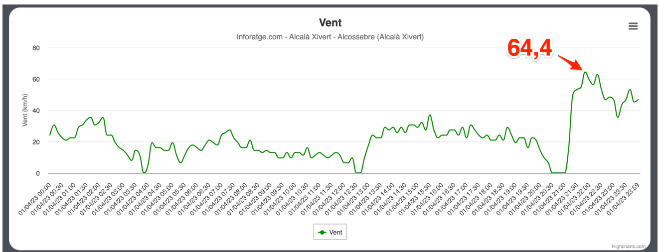
Ráfagas de viento registradas en ALCALÀ DE XIVERT el 1 de abril del 2023 https://inforatge.com/meteo-alcalaxivert
