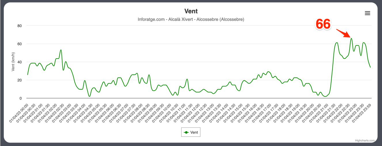
Ráfagas de viento registradas en ALCOSSEBRE el 1 de abril del 2023 https://inforatge.com/meteo-alcalaxivert
